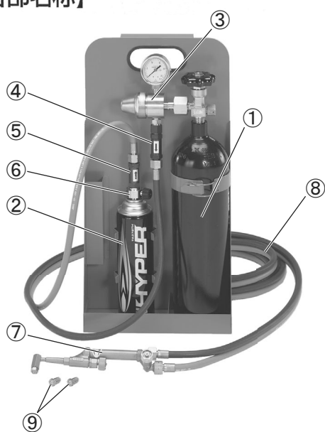
TA370TC-N
